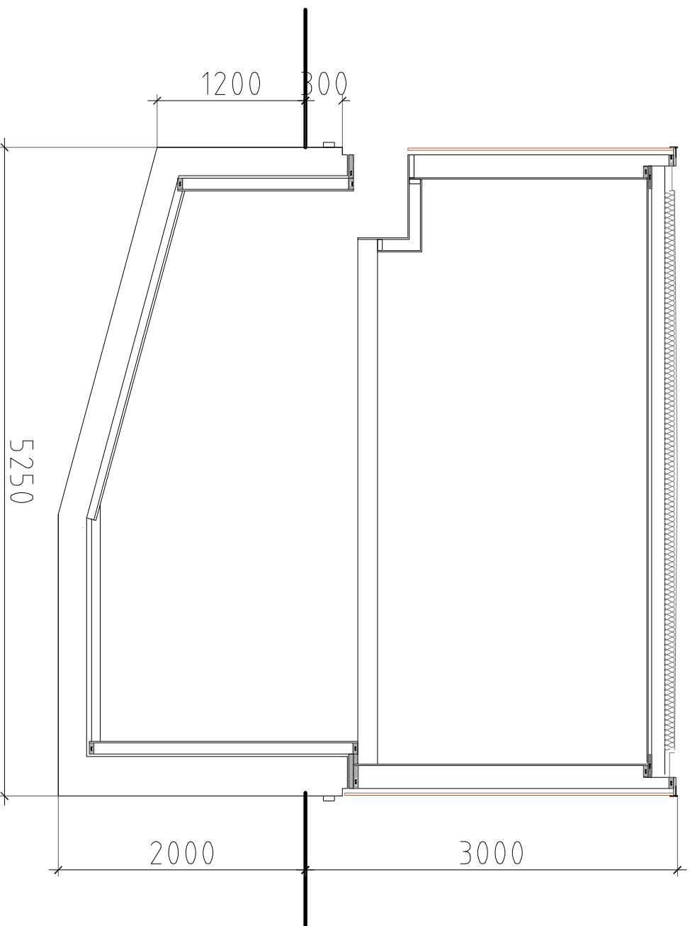
dwarsdoorsnede
